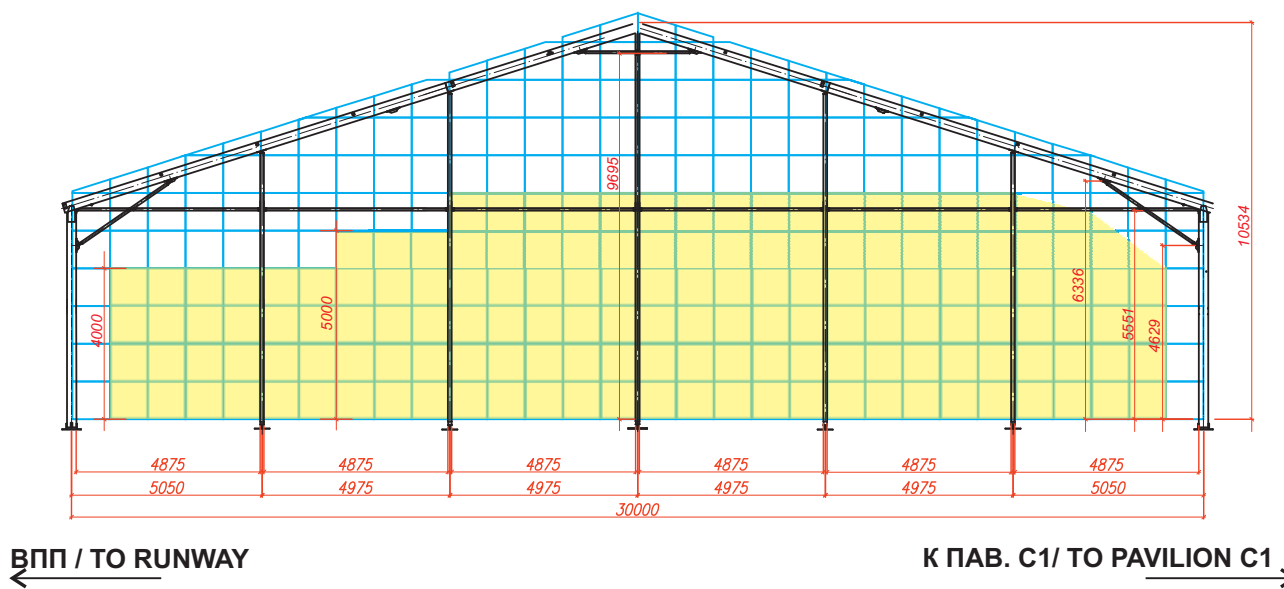
ТОРЦЕВОЙ РАЗРЕЗ ПАВИЛЬОНА D2/ CROSS SECTIONAL VIEW OF PAVILION D2
